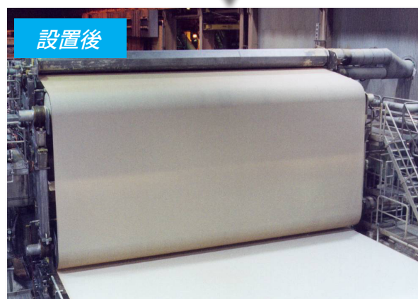
ワイヤ幅 8130mmLWC マシン、1100m/min にて運転
